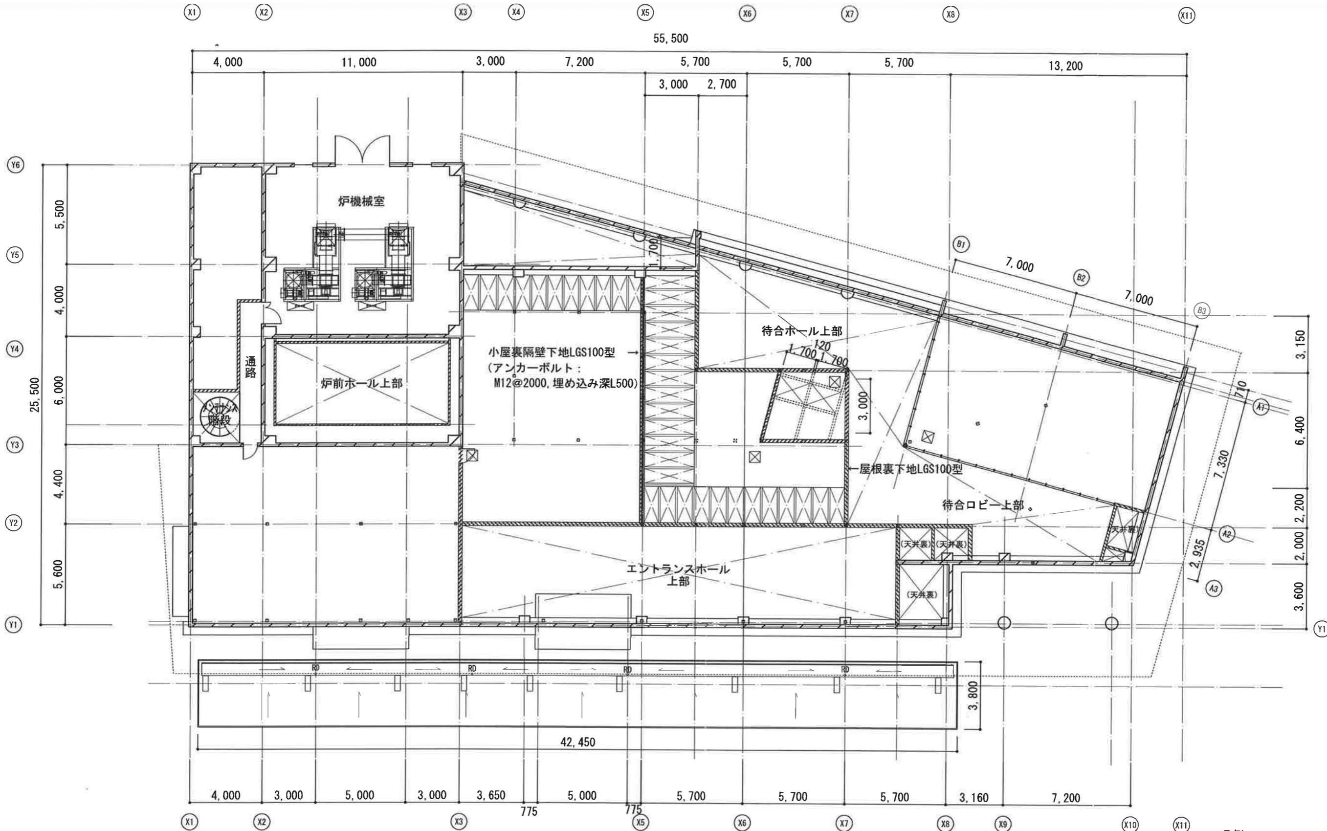
PH階1平面図
